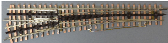
Zahnstangenweiche H0 Code 100 System Fleischmann Geometrie 6080
