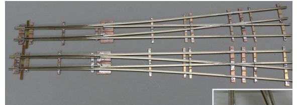
H0 EW 190 1:9 Rillenprofil Swedtram für Ladestraße
