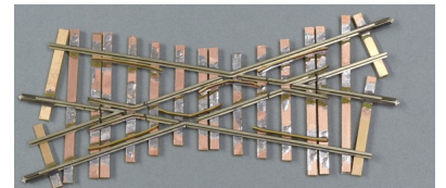
mehrspurige Weichen/Kreuzungen
