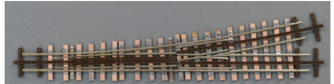
H0e Code 55 EW links r 600 / 12° Zahnstangen System Riggerbach (HFR)
